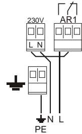
Verbraucher 230V~
